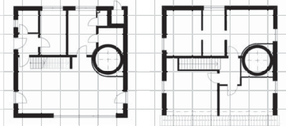
Beispielgrundriss
